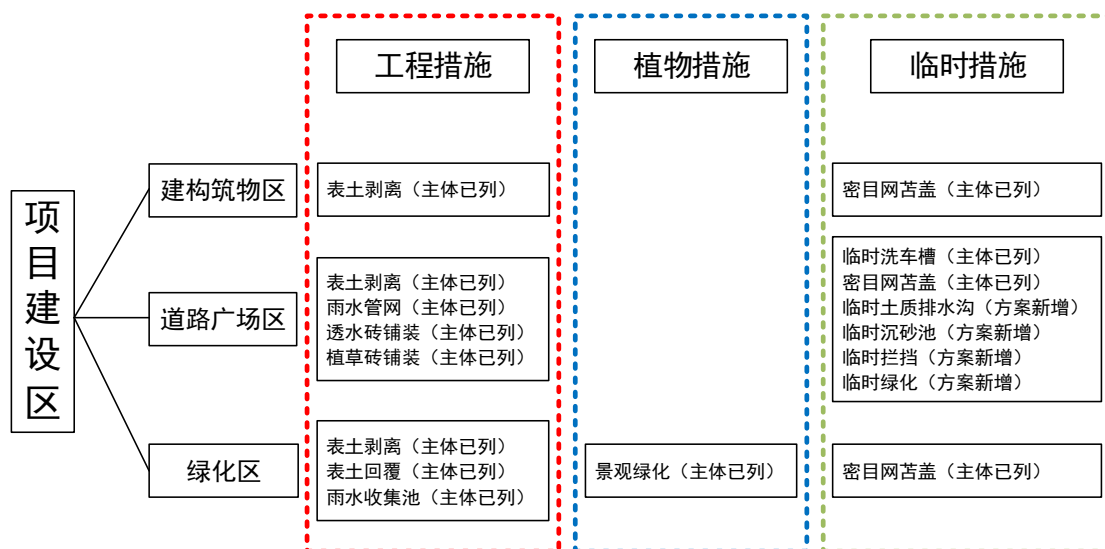
图 5-1 项目区具体措施布设体系图
