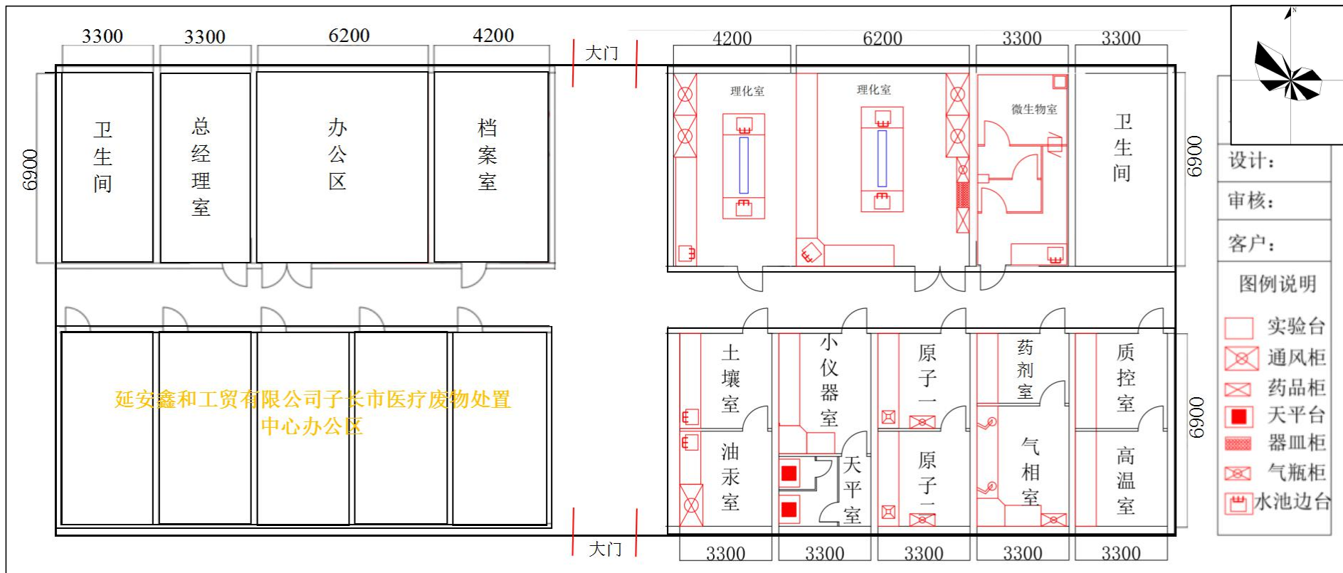
附图4 本项目平面布置图
